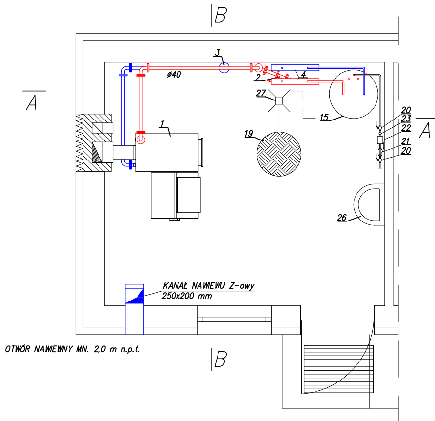
RZUT KOTŁOWNI
