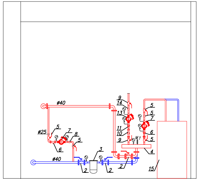
RZUT KOTŁOWNI
